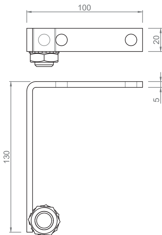
Support conducteur pose plafond
