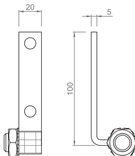
Support conducteur pose de face
